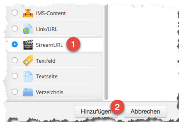
Abbildung 3: StreamURL hinzufügen
